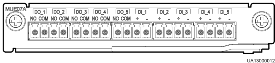
图4-19 干接点扩展卡面板示意图
