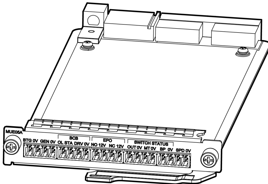
图4-15 干接点卡面板示意图
