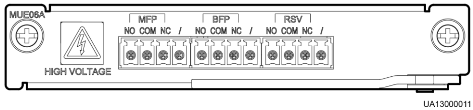
图4-18 反灌保护卡面板示意图
