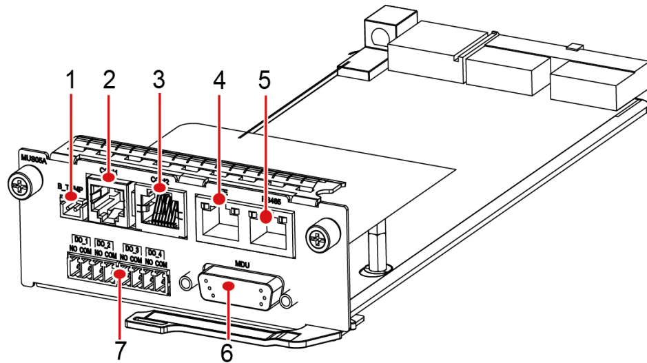
图4-16 监控接口卡面板示意图
