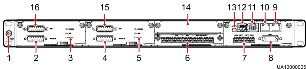
图4-11 控制模块各接口示意图
