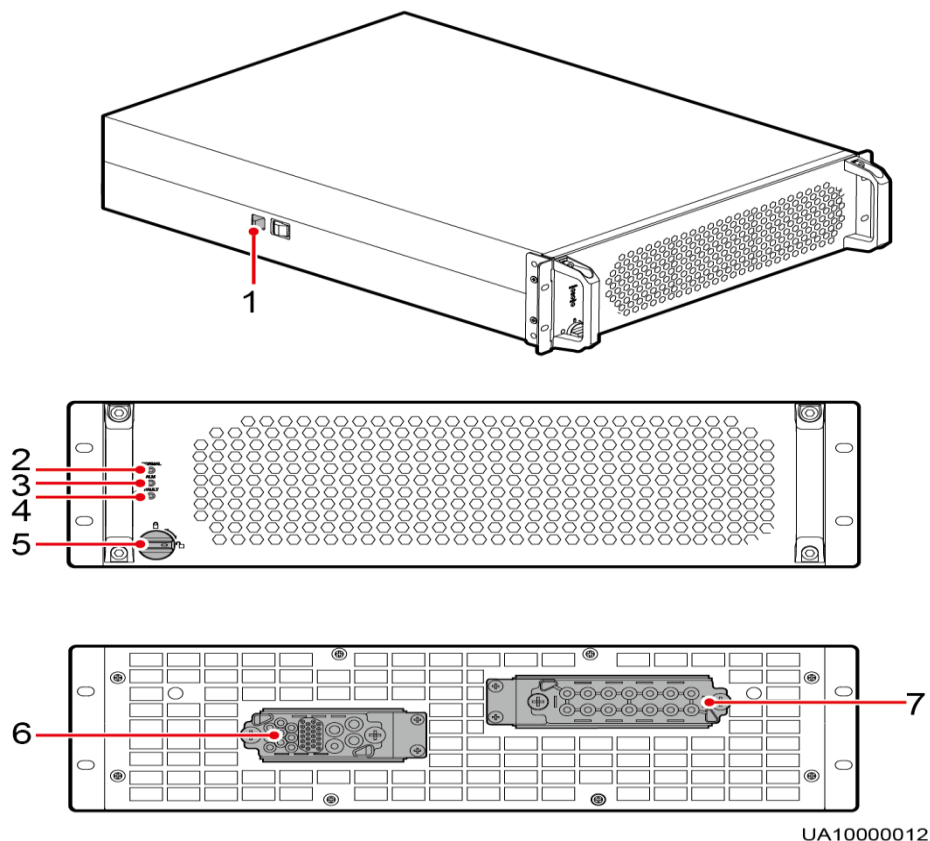
图4-7 功率模块外观示意图
