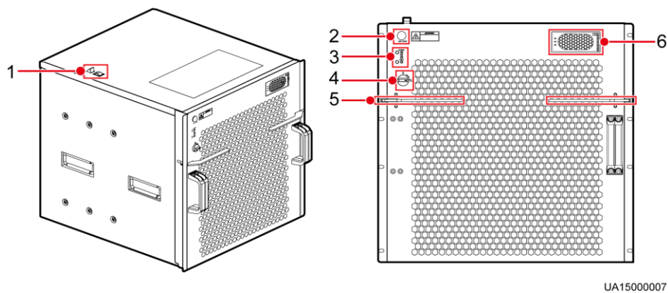
图4-9 800kVA 旁路模块外观
