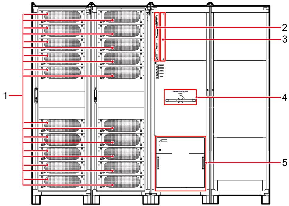
图4-5 800kVA 产品结构（标配版）
