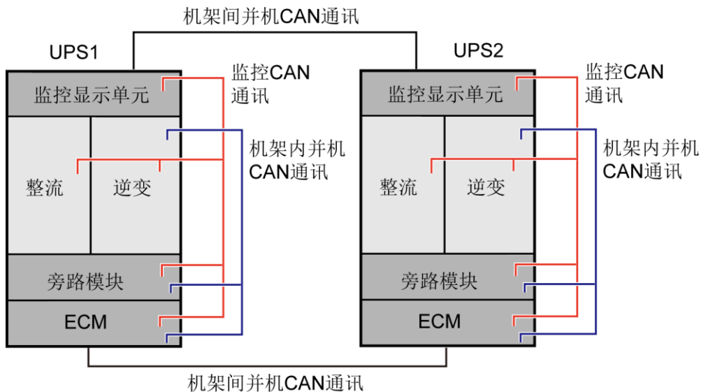
图4-14 CAN 通讯逻辑示意图
