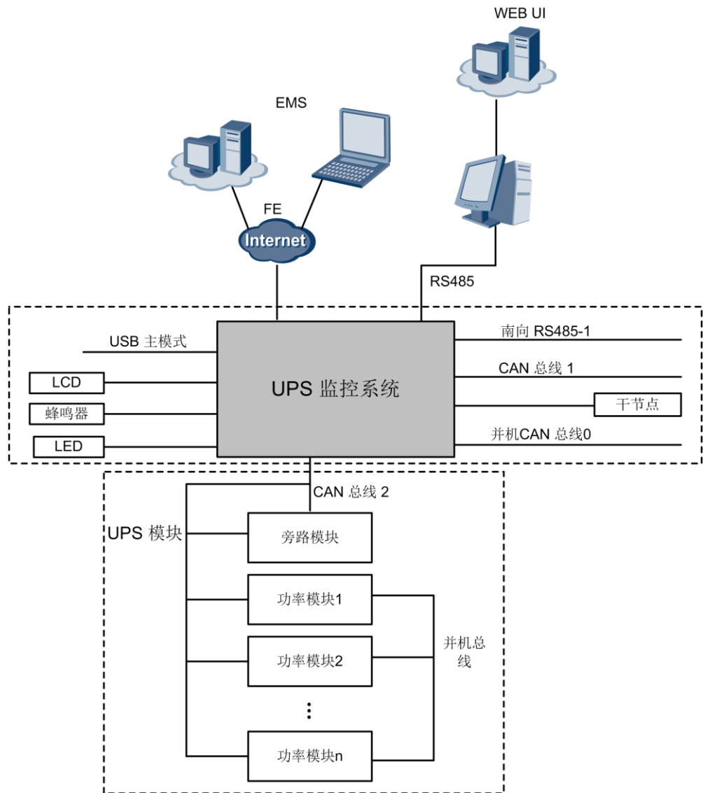
图4-12 监控单元系统在 UPS5000-E 系统中的示意图
