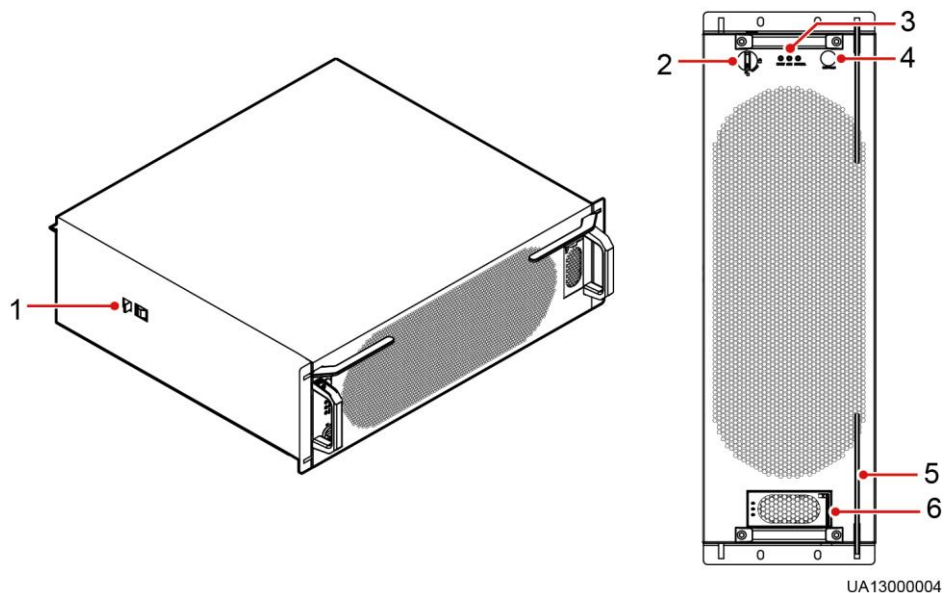
图4-8 600kVA 旁路模块外观
