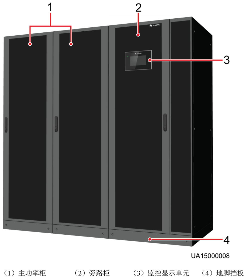
图4-1 UPS5000-E-600kVA 外观
