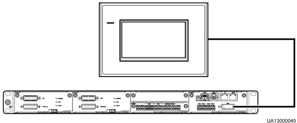
图4-10 UPS5000-E 监控单元系统示意图
