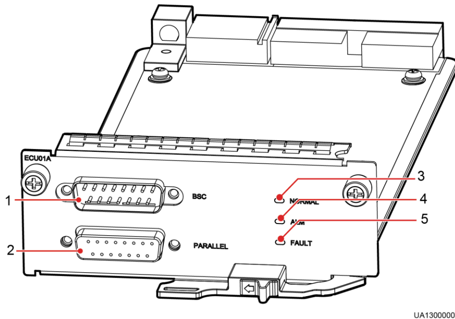
图4-13 ECM 面板示意图
